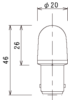
BA 15 d 口金
