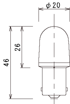
BA 15 s 口金
